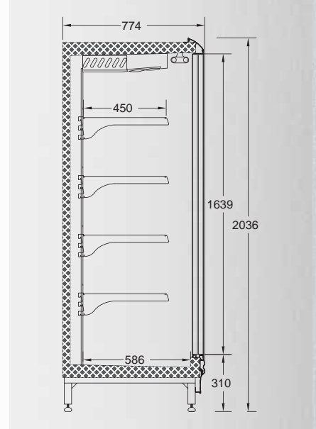
Çiğdem Sürgülü / Crocus Sliding Door
